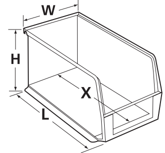
Guía de Dimensiones L (longitud), W (ancho), H (altura), X (longitud interior)
